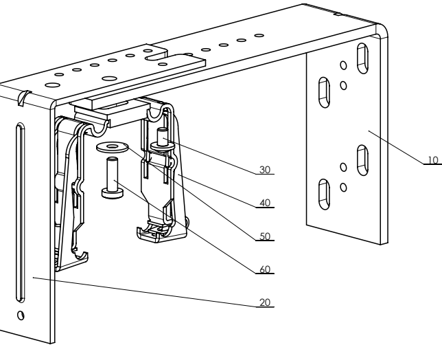
Doppio supporto regolabile - meccanico 306 – 368 mm P 010/41 (2-01799-0000)
