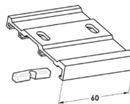
Supporto del profilo superiore (6-009232)
