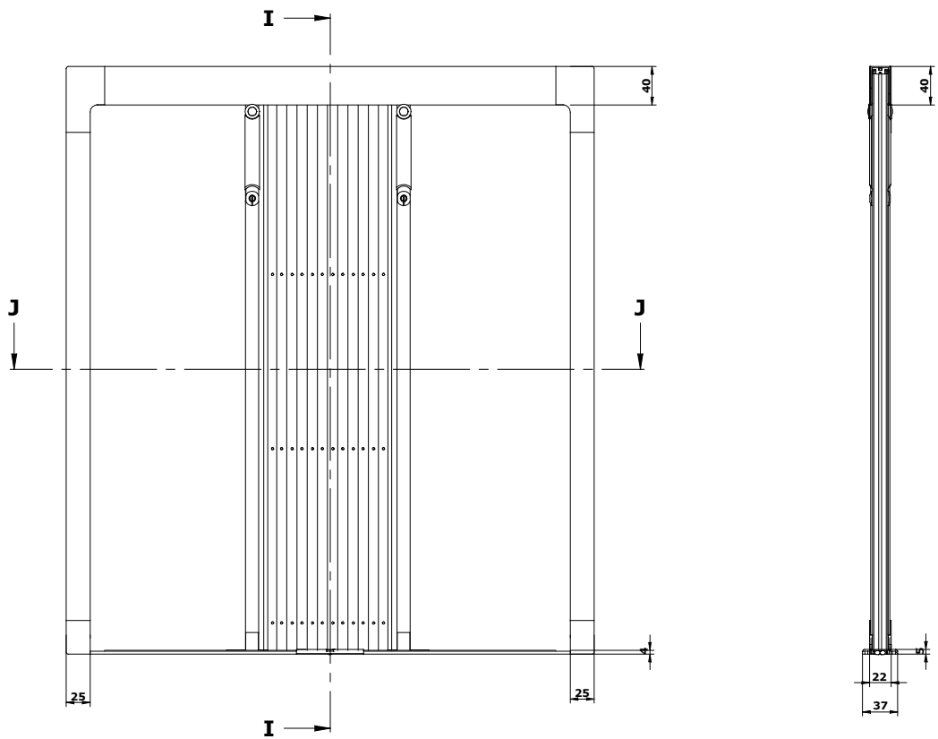
SEZIONE I-I
