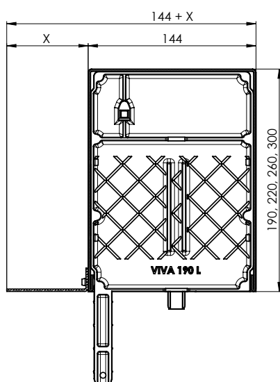
Sezione cassonetto a muro VIVA + P 020/07-20, P 080/07-20, P 081/07-20 190 x 140b 220 x 140b 260 x 140b 300 x 140b
