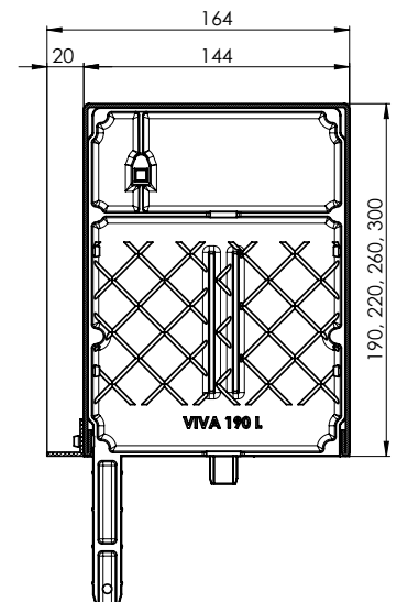
Sezione cassonetto a muro VIVA + P 020/02, P 080/02, P 081/02 190 x 140b 220 x 140b 260 x 140b 300 x 140b
