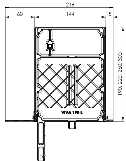
Sezione cassonetto sotto intonaco VIVA + P 020/06, P 080/06, P 081/06 190 x 150Lb 220 x 150Lb 260 x 150Lb 300 x 150Lb
