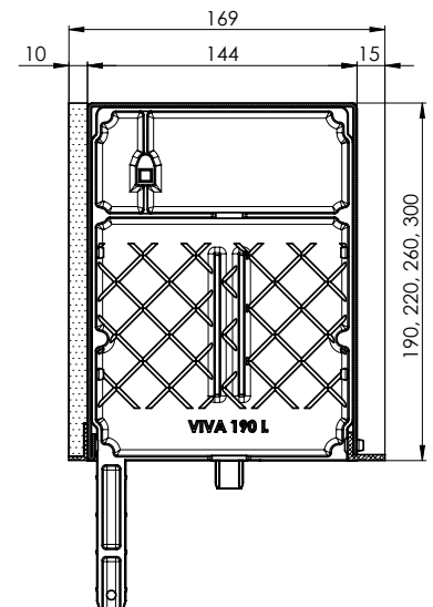
Sezione cassonetto sotto intonaco VIVA 190 x 169 x 2L x STY10 220 x 169 x 2L x STY10 260 x 169 x 2L x STY10 300 x 169 x 2L x STY10
