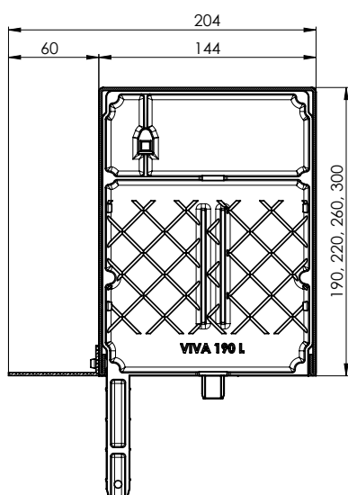
Sezione cassonetto a muro VIVA + P 020/06, P 080/06, P 081/06 190 x 140b 220 x 140b 260 x 140b 300 x 140b
