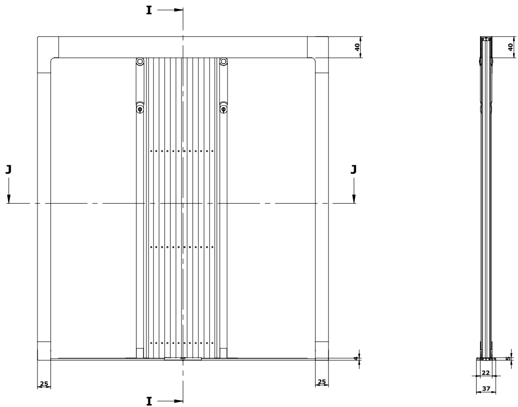
SEZIONE I-I
