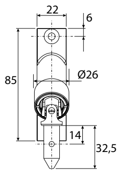
Snodo cardanico 90°
