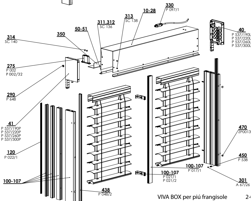
CASELLA PER LA FRANGISOLE ESTERNA AUTOPORTANTE (lista di guida P 080) 2-01016-XXXX-D
