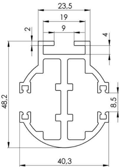
Lista di guida rotonda doppia P 017/7 (7-302155)
