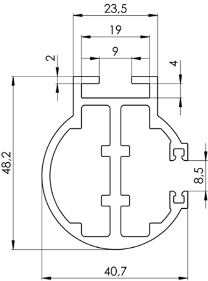
Lista di guida rotonda semplice P 018/7 (7-302154)
