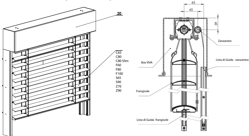
FRANGISOLE ESTERNA AUTOPORTANTE 2-01010-0000-B
