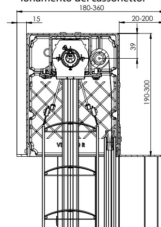
Taglio di Frangisole autoportante intonato Viva (Profili di estensione utilizzati) Preparato per il polistirene dal lato frontale)
